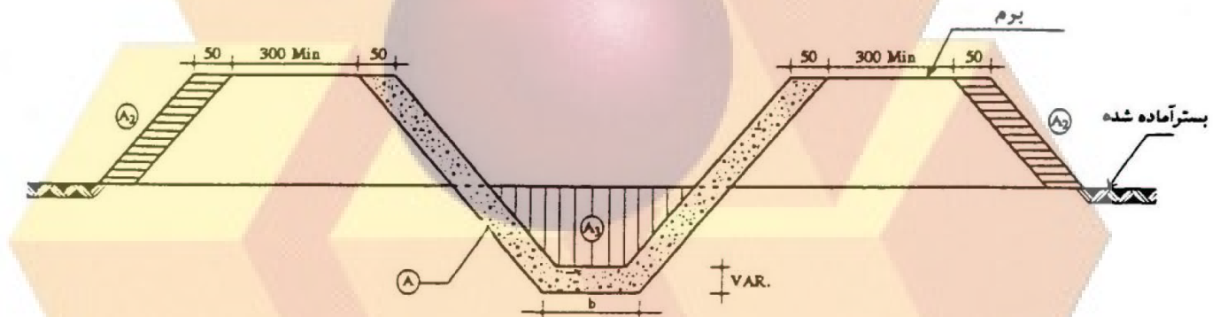
شکل ۳-۵. شمای مقطع خاکبرداری
